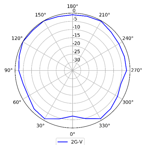
2.4GHz (Vertical)
