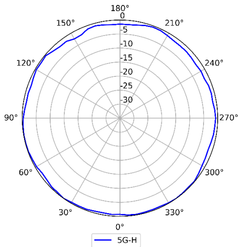
5GHz (Horizontal)
